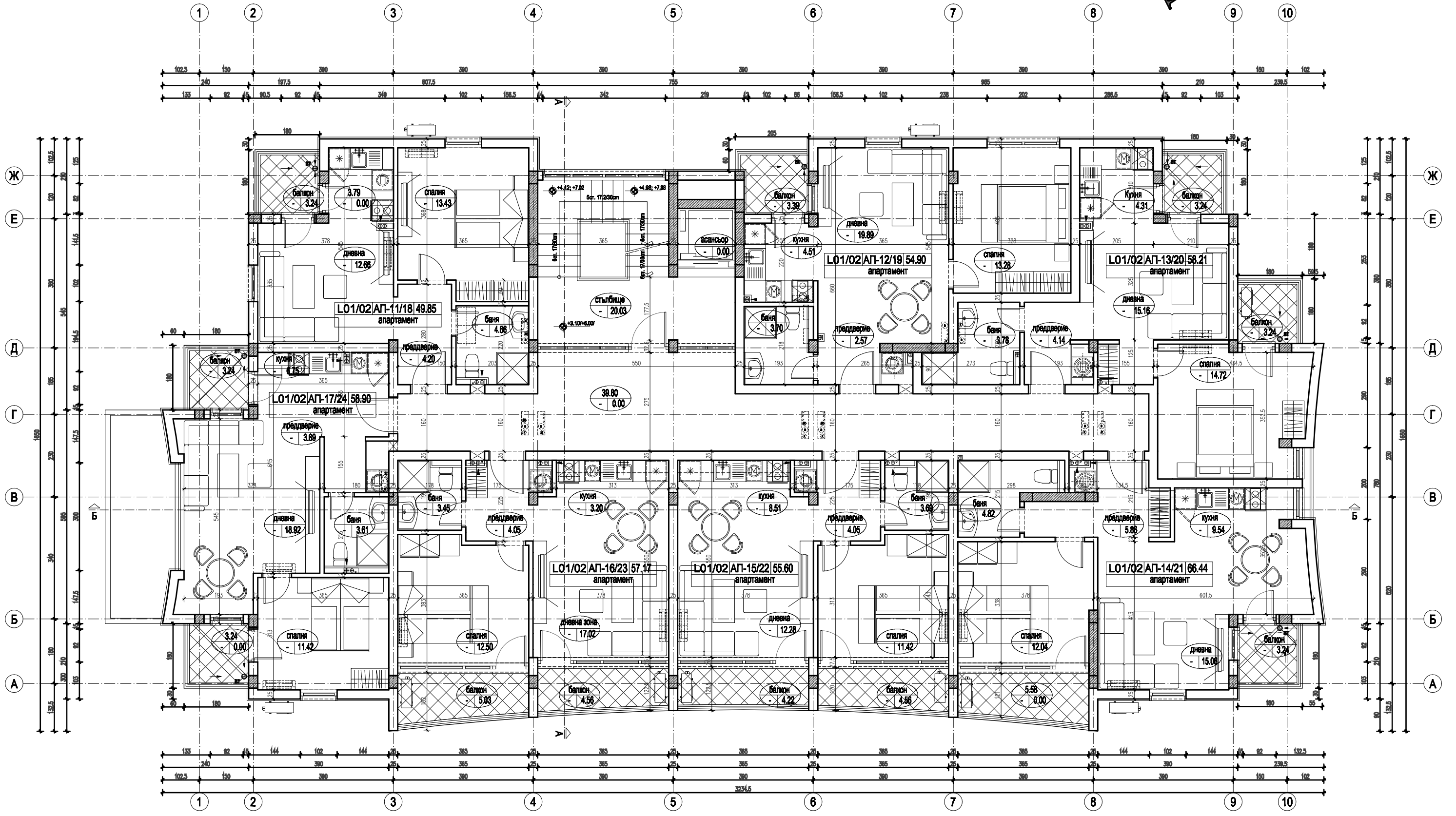
РАЗПРЕДЕЛЕНИЕ КОТИ +3.10; +6.00 М 1:50 ЗАСТРОЕНА РЕАЛНА ПЛОЩ ЕТАЖИ II-ри ; III-ти = 475.20 м²
