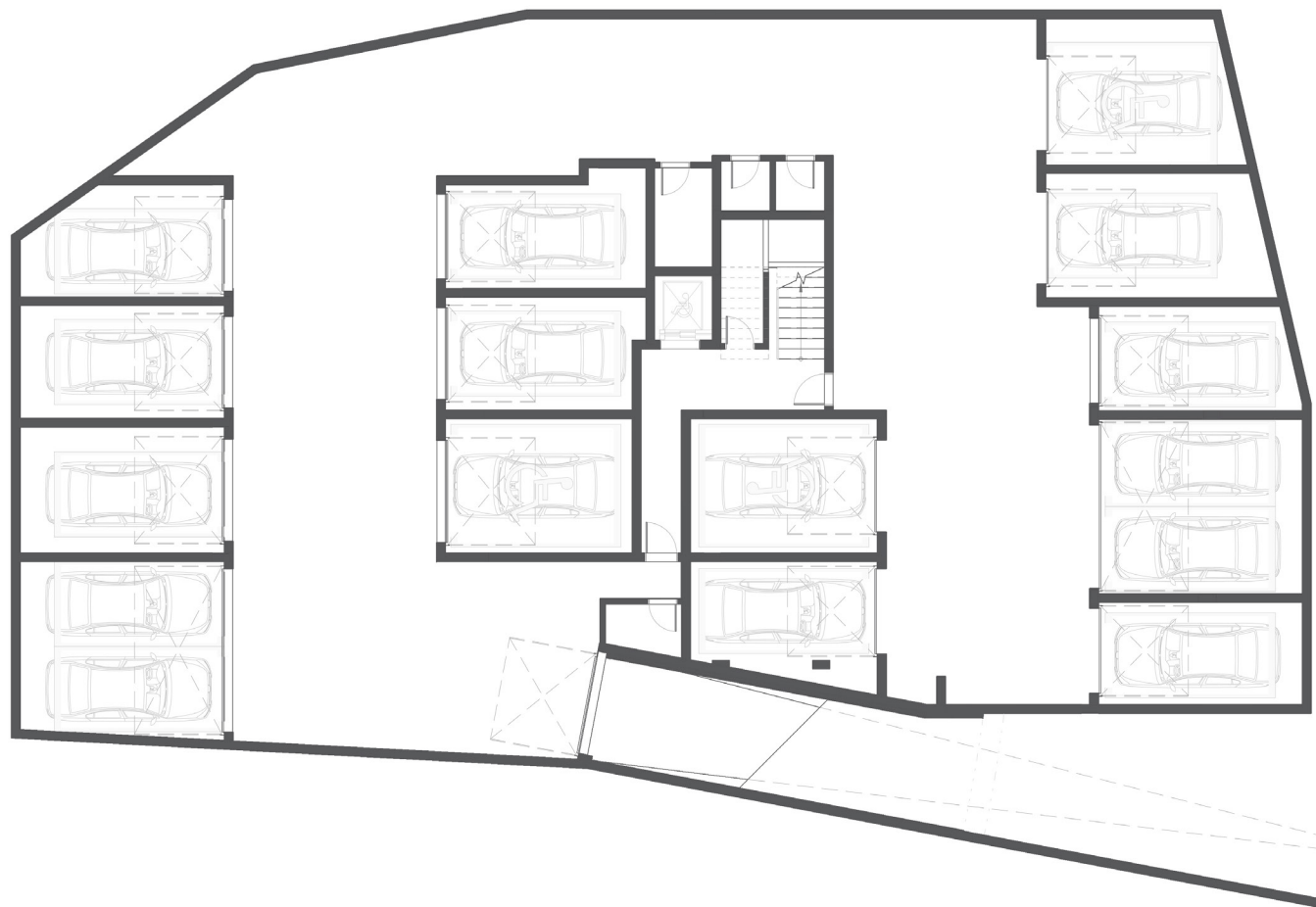
РАЗПРЕДЕЛЕНИЕ КОТА -3.30
